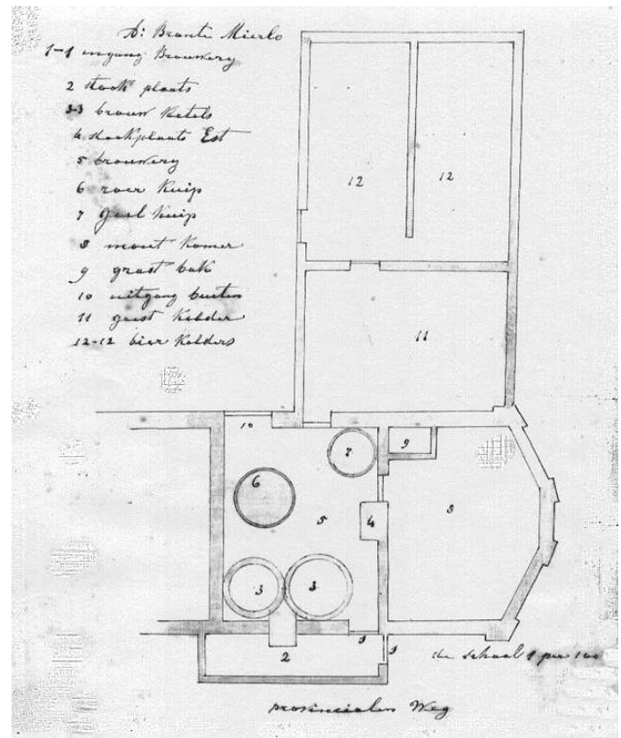
Plattegrond van brouwerij het Vertrouwen aan de Dorpsstraat met o.a. 2=stookplaats, 3=brouwketels, 8=moutkamer, 11=gerstkelder, 12=bierkelders.
